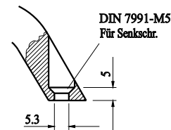
Frontseitige Befestigung
