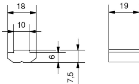
Nutenstein einschiebbar ohne Positionierung
