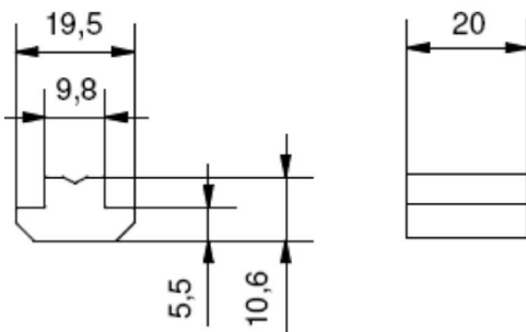
Nutenstein schwer ohne Positionierung
