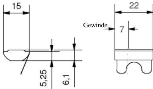
Nutenstein einschenkbar mit Positionierung
